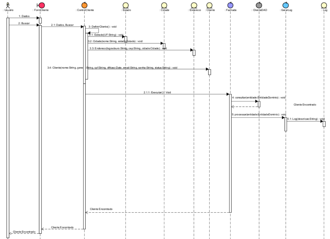
Figura 12 - Buscar Cliente.
