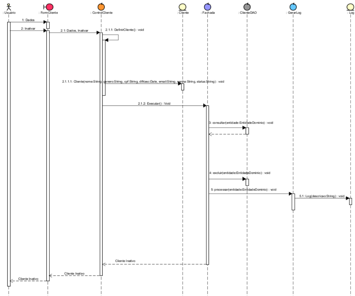
Figura 14 - Inativar Cliente.
