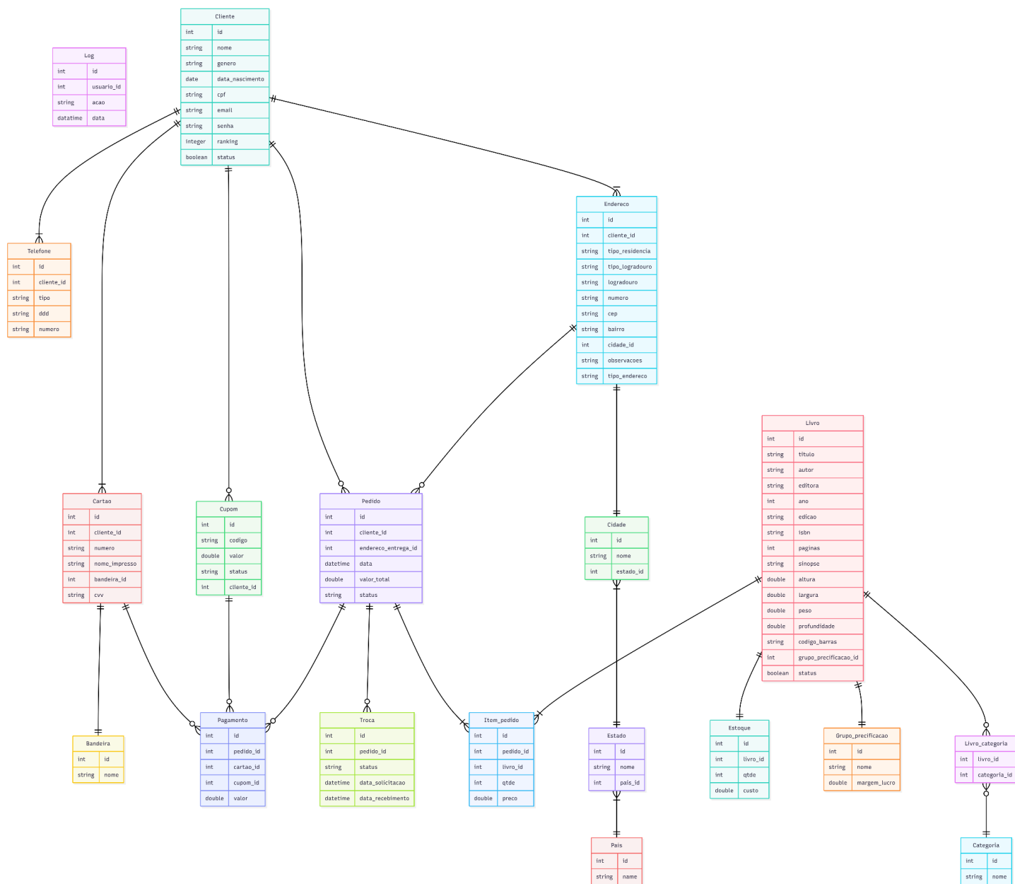
Figura 17– Modelo Físico
