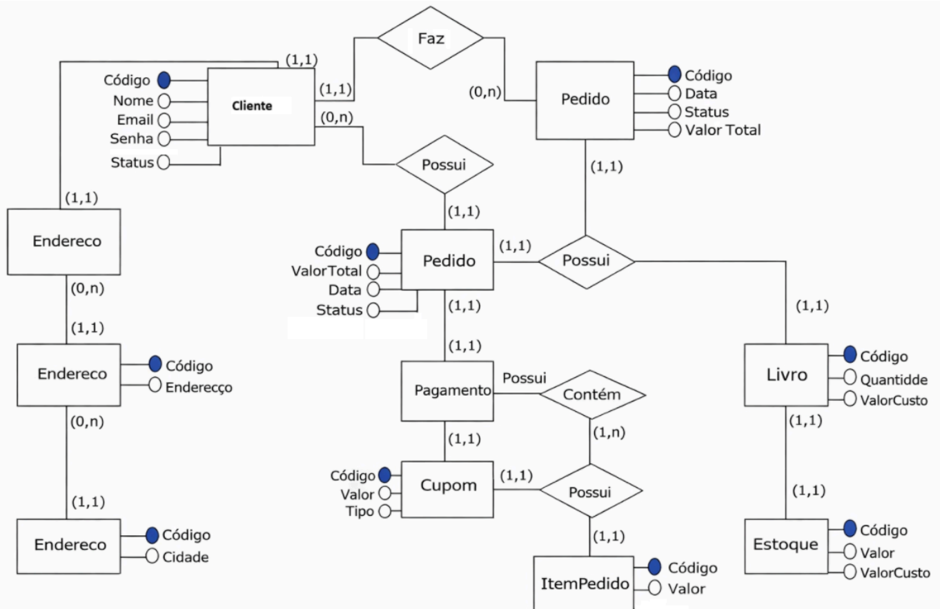
Figura 16– Modelo Lógico
